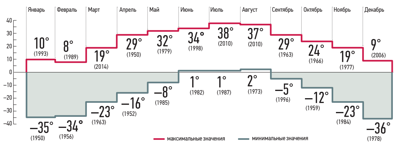
Минимумы и максимумы среднемесячной температуры в Москве (в градусах Цельсия)
