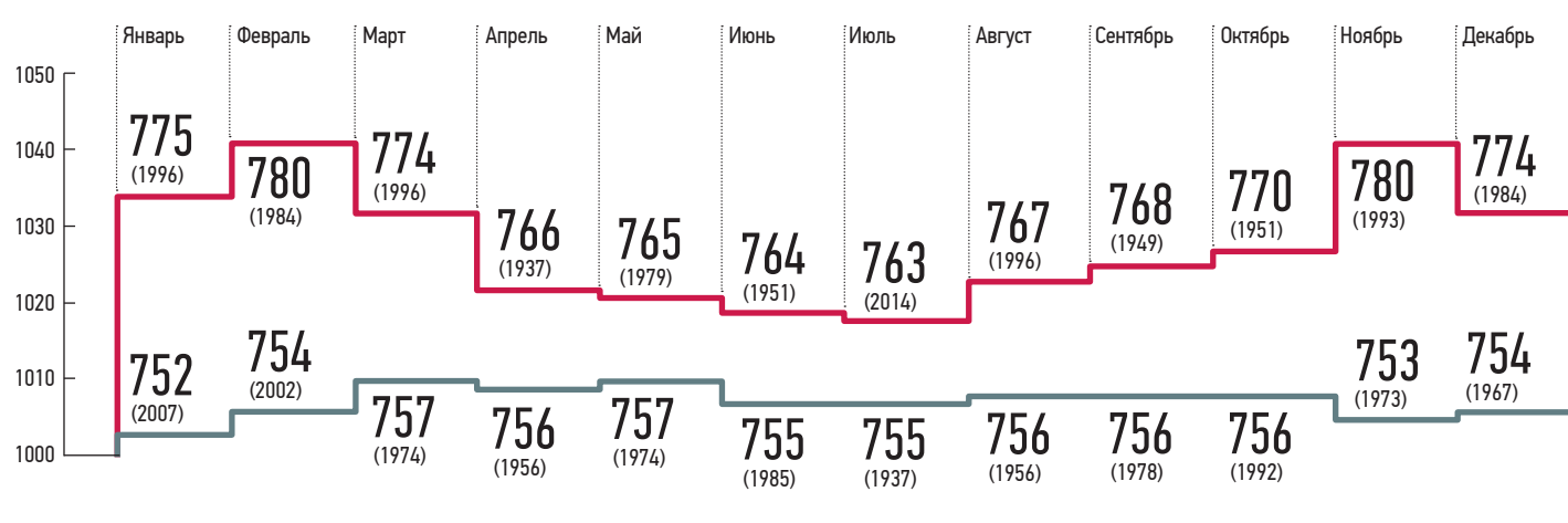
Минимумы и максимумы среднемесячного атмосферного давления в Москве (мм рт. ст.)
