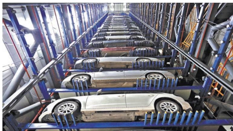
Этот гараж в китайском Хучжоу позволяет на площади 49 кв. метров вместить до 50 автомобилей. Секрет — высота гаража в 25 этажей.
