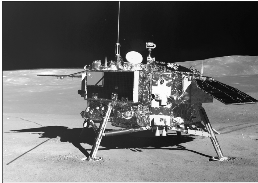
Лунный зонд «Чанъэ-4» успешно выполнил свою миссию. Фото: Китайское национальное космическое управление (Синьхуа).
