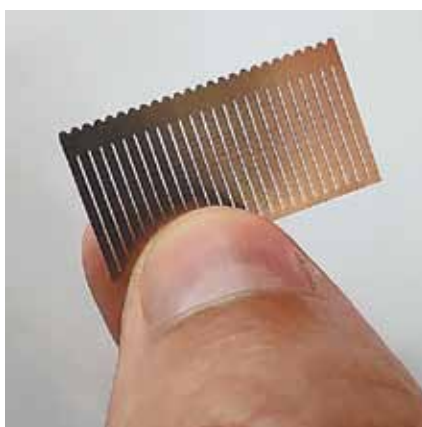
Пружина из БрБ2 0,2 мм
