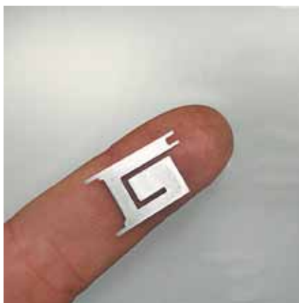
Антенна из нержавеющей стали 0,3 мм
